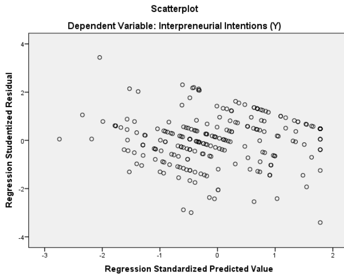
Gambar 1. Grafik Scatterplot
